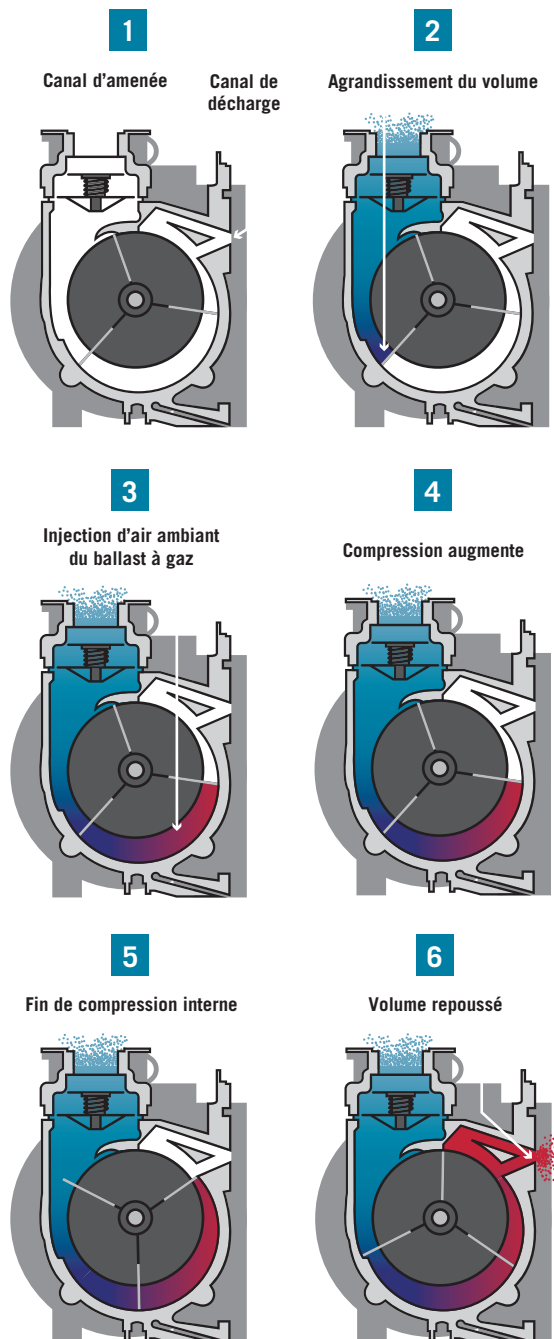
Processus de chambre de compression de pompe à vide à palettes rotatives.
